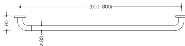
Dimensioner i mm
