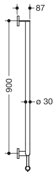
Dimensioner i mm
