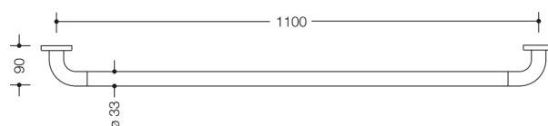
Dimensioner i mm
