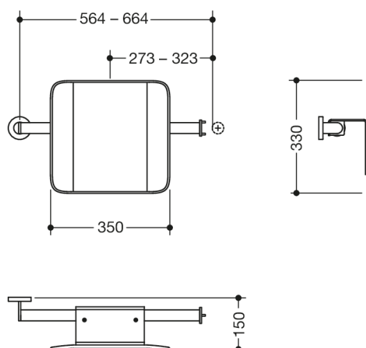
Dimensioner i mm
