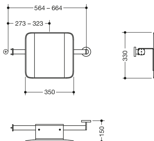
Dimensioner i mm
