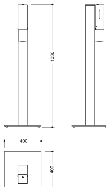
Dimensioner i mm
