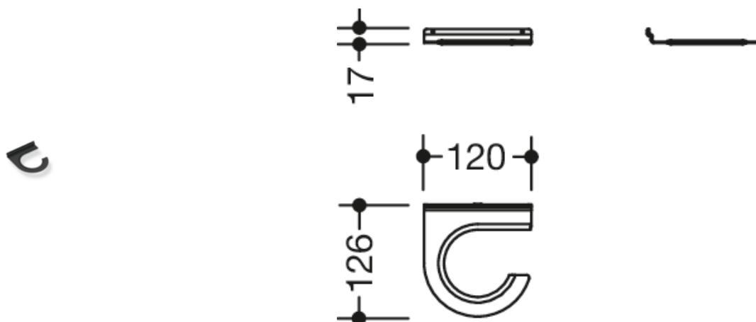
Dimensioner i mm
