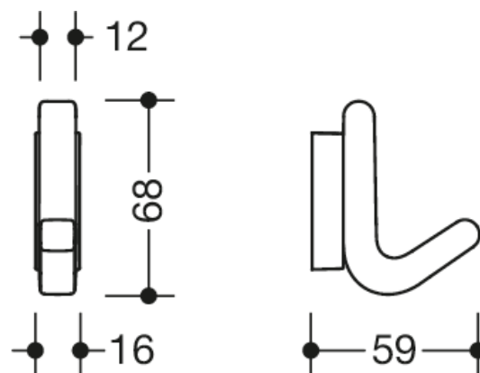
Dimensioner i mm
