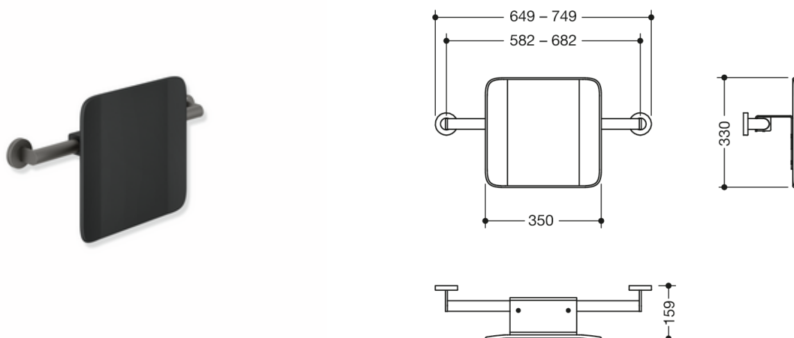
Dimensioner i mm
