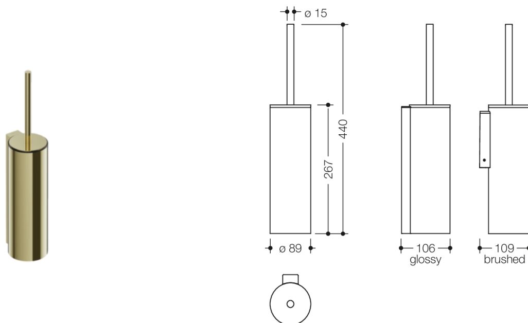
Dimensioner i mm
