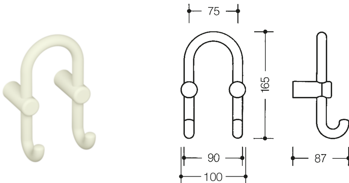
Dimensioner i mm
