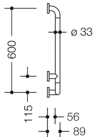
Dimensioner i mm
