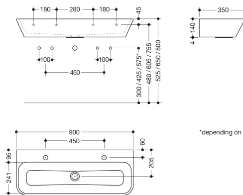
Dimensioner i mm
