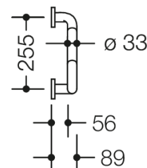
Mesures en mm
