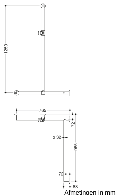
Afmetingen in mm
