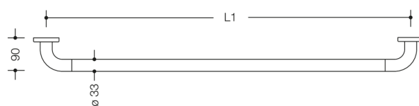
Afmetingen in mm
