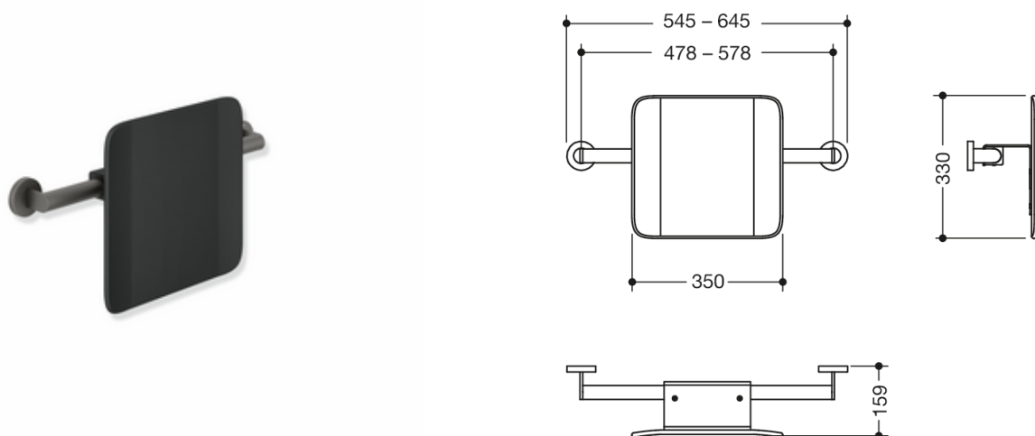
Afmetingen in mm
