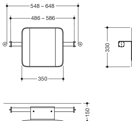
Afmetingen in mm
