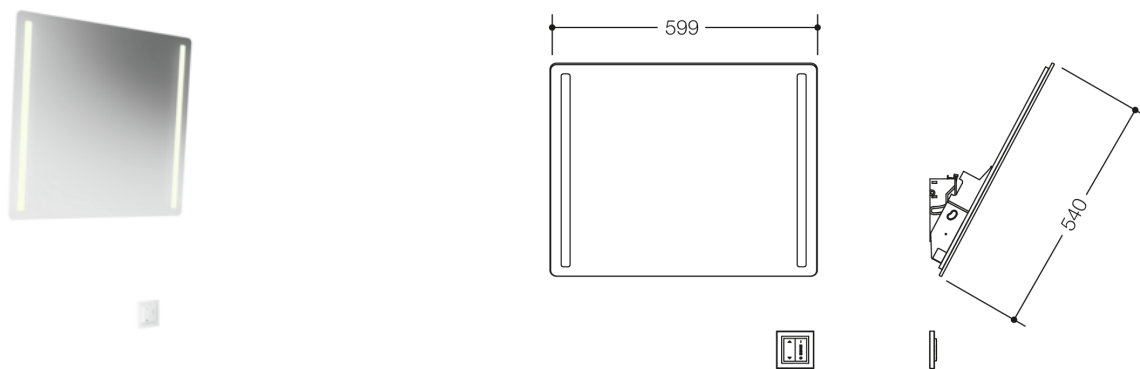
Afmetingen in mm
