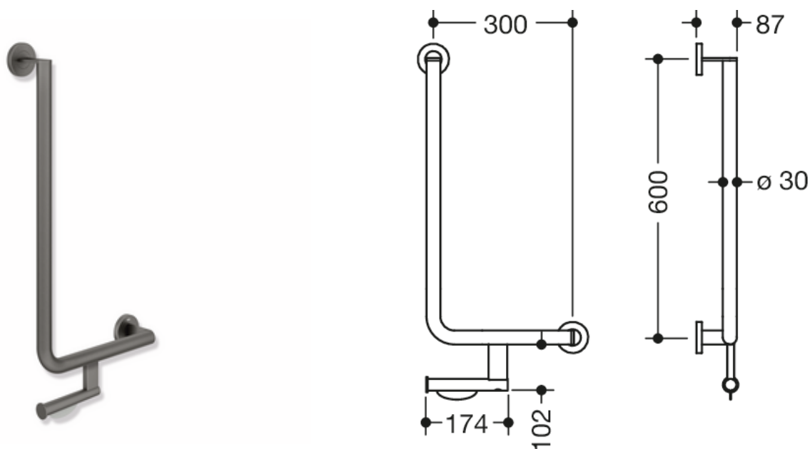
Afmetingen in mm
