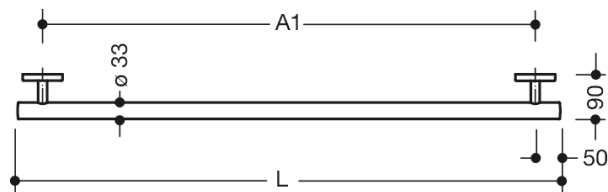
Afmetingen in mm
