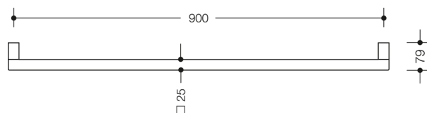
Dimensjoner i mm
