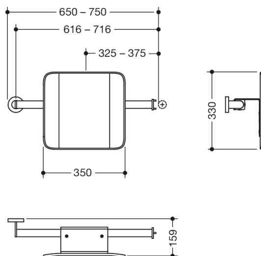
Dimensjoner i mm
