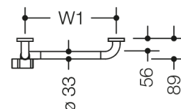
Dimensjoner i mm
