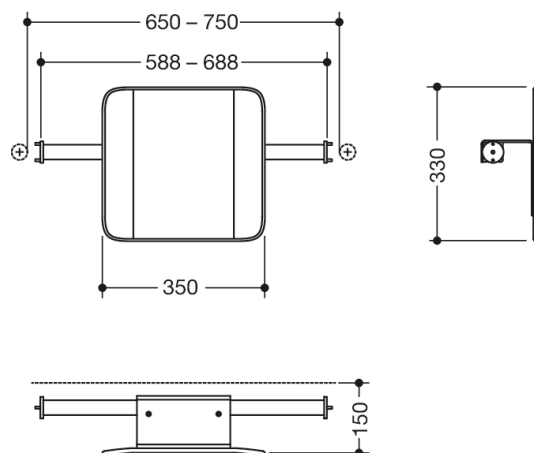
Dimensjoner i mm
