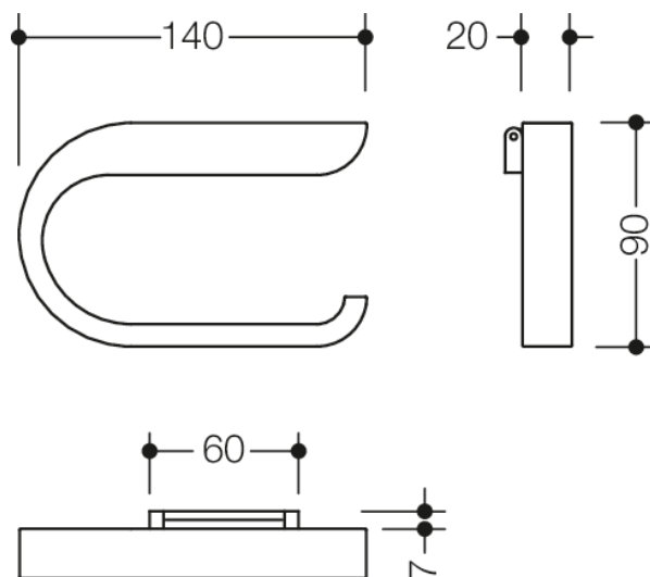
Dimensjoner i mm
