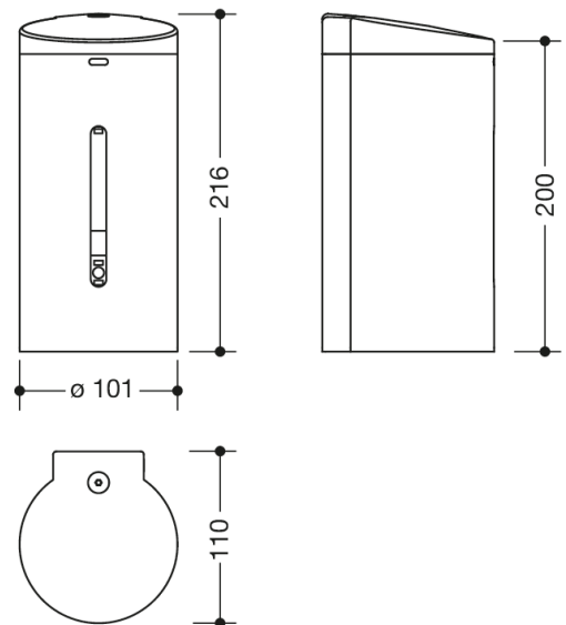
Dimensjoner i mm
