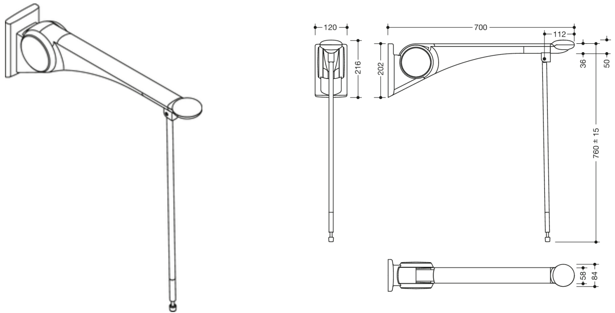
Dimensjoner i mm
