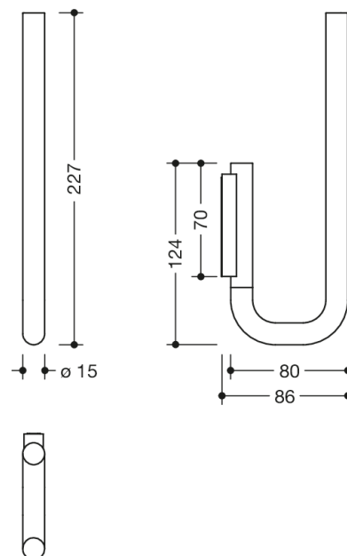
Dimensjoner i mm
