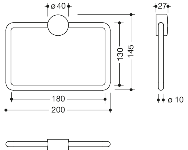
Dimensjoner i mm
