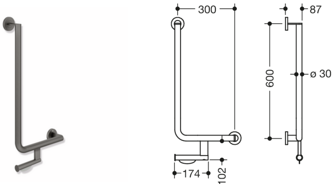
Dimensjoner i mm
