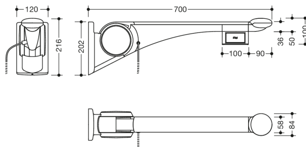
Dimensjoner i mm
