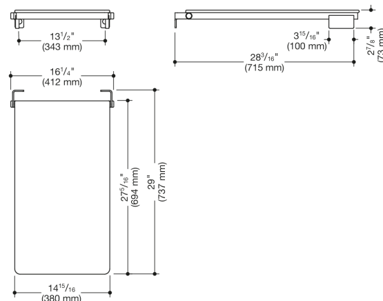
Dimensjoner i mm
