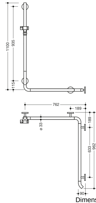
Dimensjoner i mm
