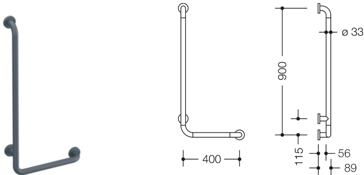
Dimensjoner i mm
