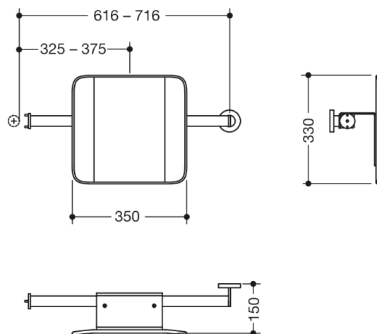
Dimensjoner i mm
