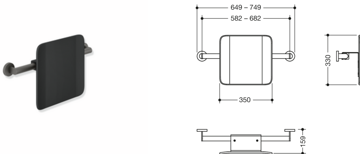
Dimensjoner i mm
