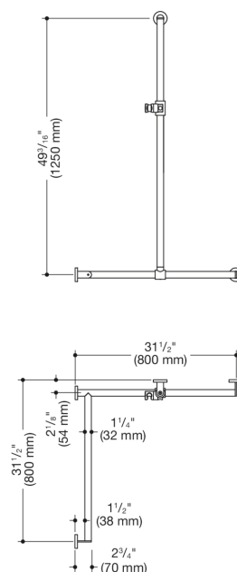
Dimensjoner i mm
