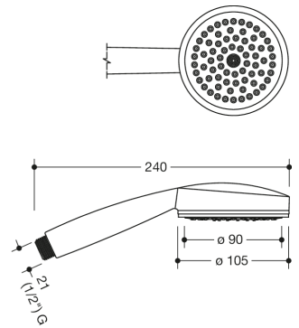
Dimensjoner i mm
