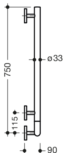
Wymiary w mm
