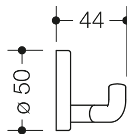
Wymiary w mm
