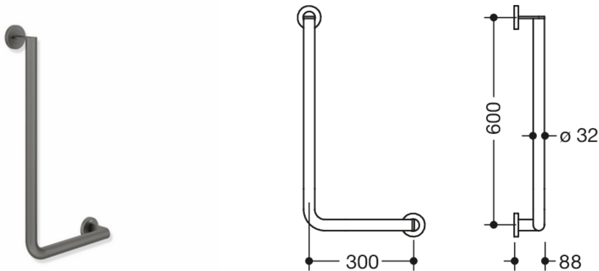
Wymiary w mm
