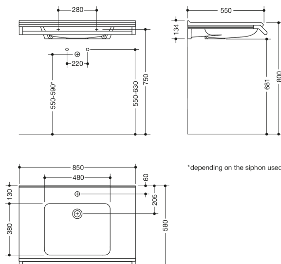
Wymiary w mm
