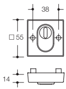
Security escutcheon 308X..ESZ
