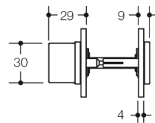
Wymiary w mm
