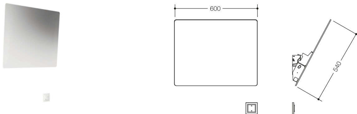
Wymiary w mm
