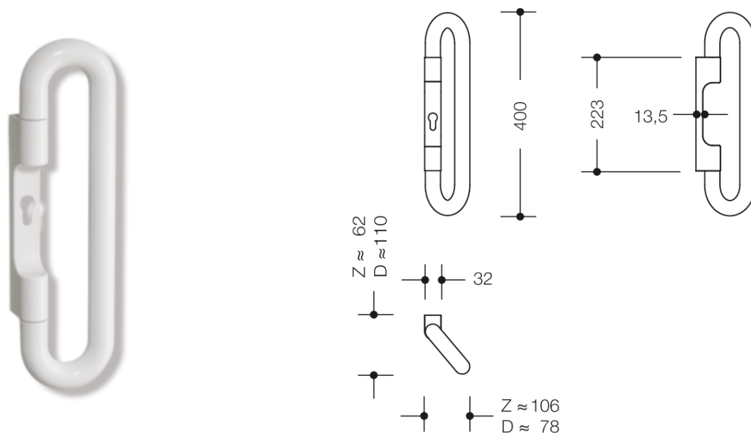
Mesures en mm
