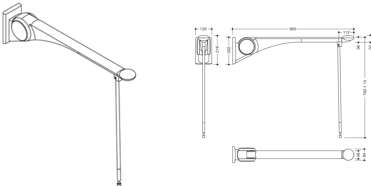
Mått i mm
