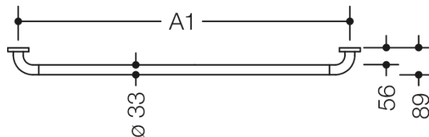
Mått i mm
